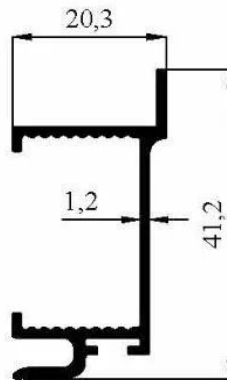
3265 0,314 kg/m
