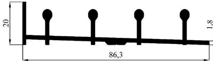
3918 0,906 kg/m
