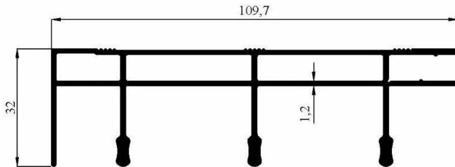
3259 1,279 kg/m
