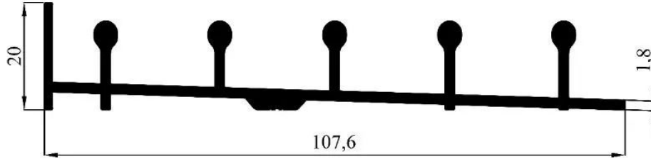
3925 1,104 kg/m
