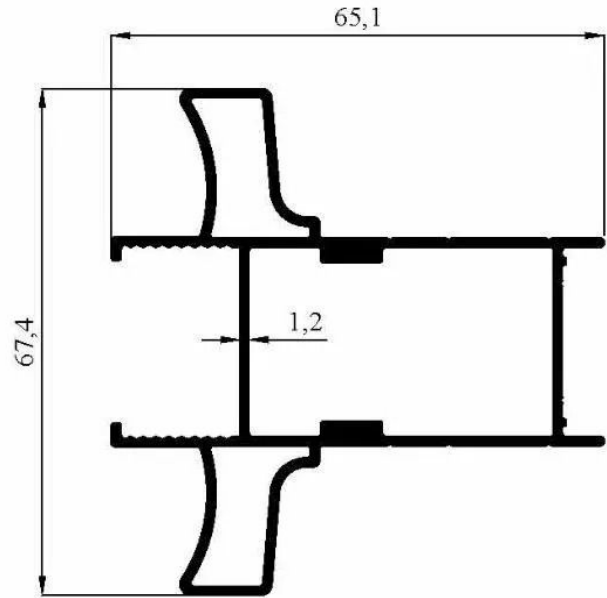
3267 1,029 kg/m
