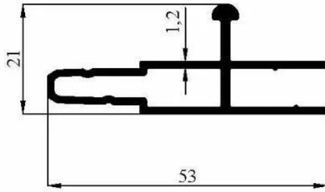
3261 0,469 kg/m
