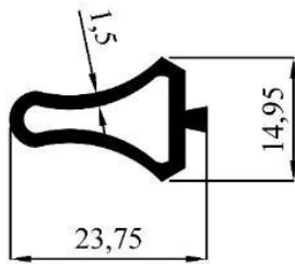
2386 0,244 kg/m
