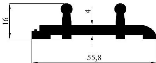
2393 0,888 kg/m
