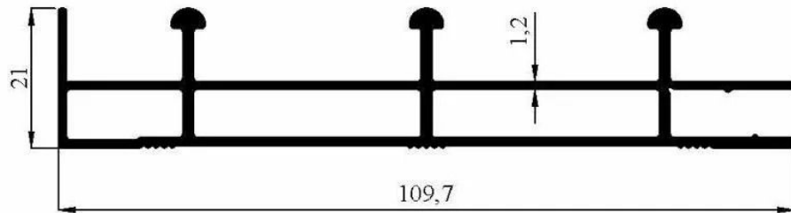
3258 1,098 kg/m
