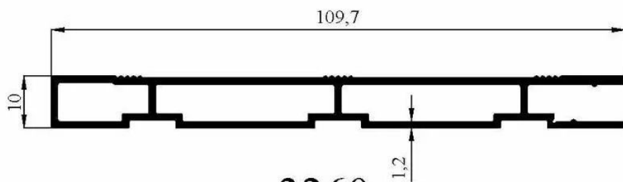
3260 0,846 kg/m
