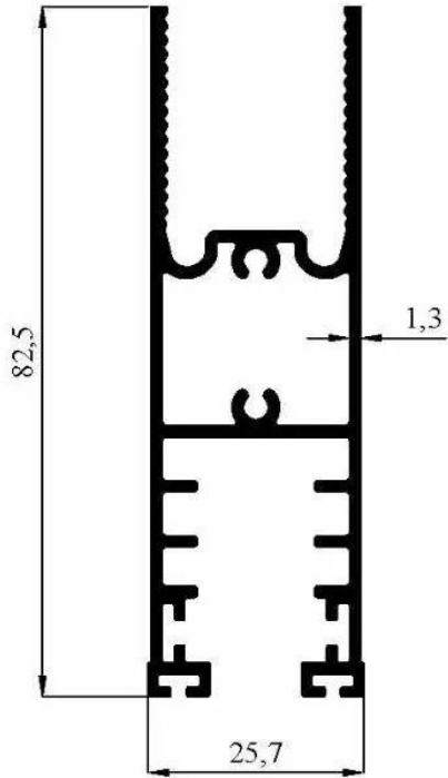
3266 1,119 kg/m
