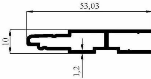
3263 0,404 kg/m
