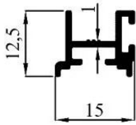
1788 0,145 kg/m
