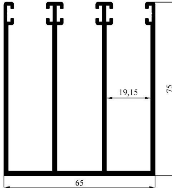
3913 1,910 kg/m
