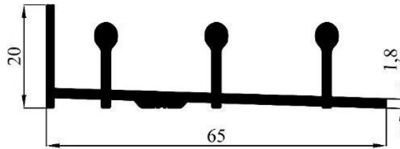
3915 0,707 kg/m
