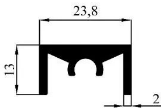
2391 0,366 kg/m
