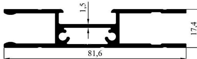
3919 0,931 kg/m
