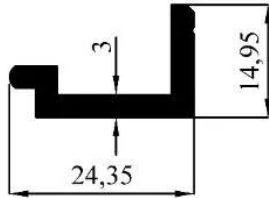
2397 0,320 kg/m
