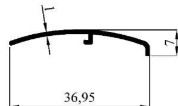
2394 0,119 kg/m
