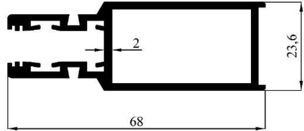
2385 0,997 kg/m
