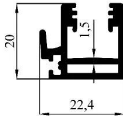
2384 0,420 kg/m
