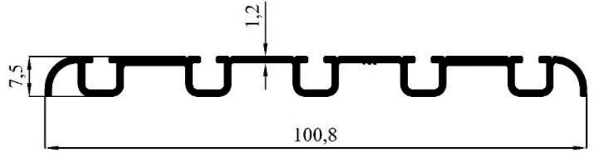
1787 0,615 kg/m
