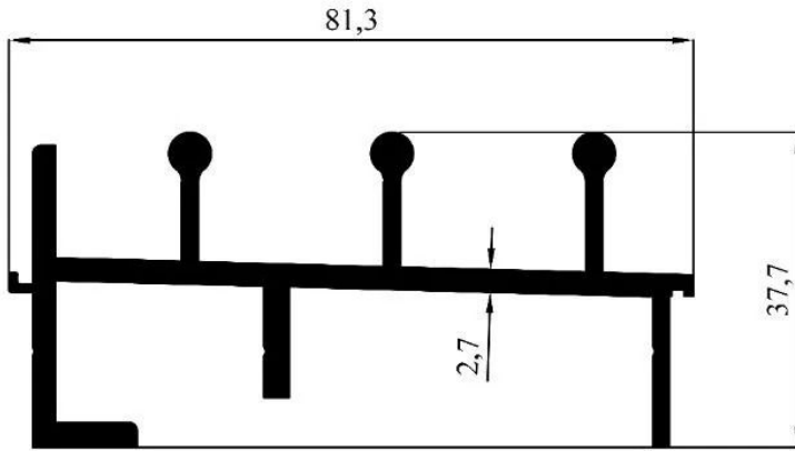
2395 1,447 kg/m
