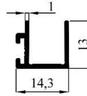
3920 0,126 kg/m
