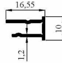
3264 0,122 kg/m
