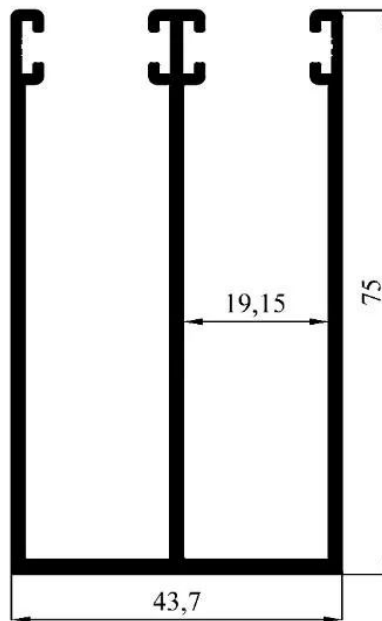
3910 1,387 kg/m
