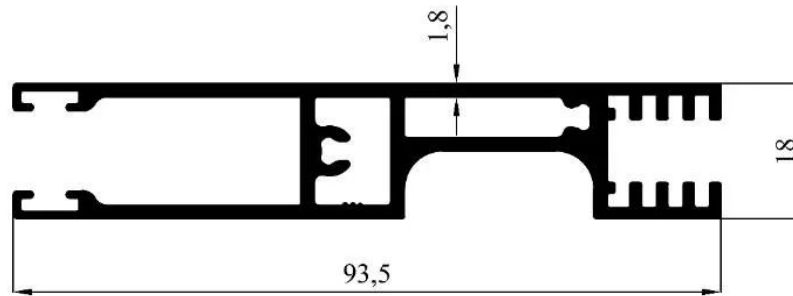
2211 1,339 kg/m
