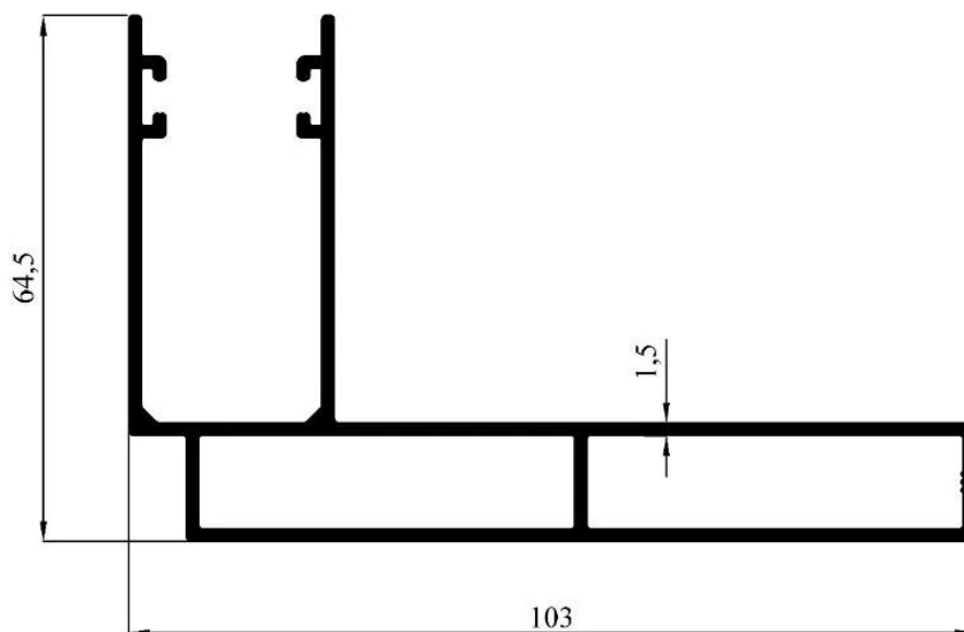
2257 1,439 kg/m
