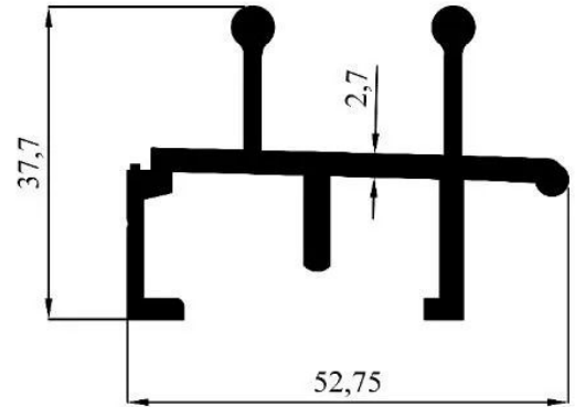
2396 1,003 kg/m
