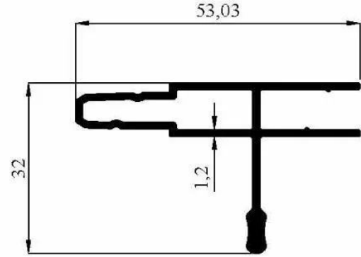
3262 0,518 kg/m
