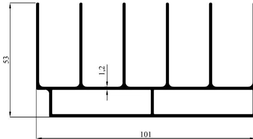
1793 1,539 kg/m
