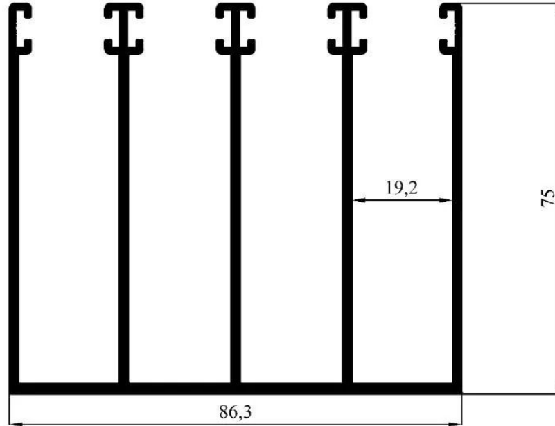
3916 2,433 kg/m
