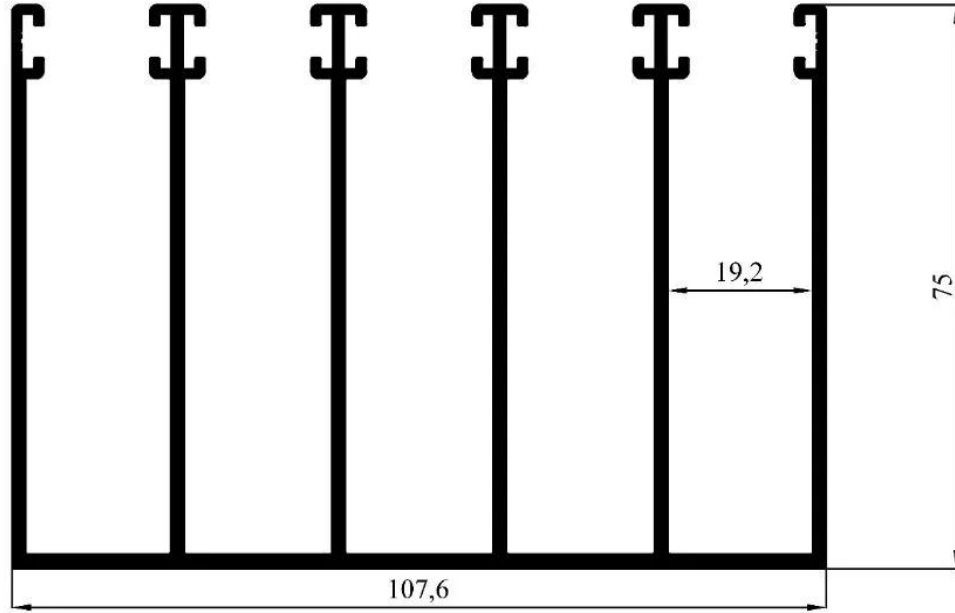
3923 2,956 kg/m
