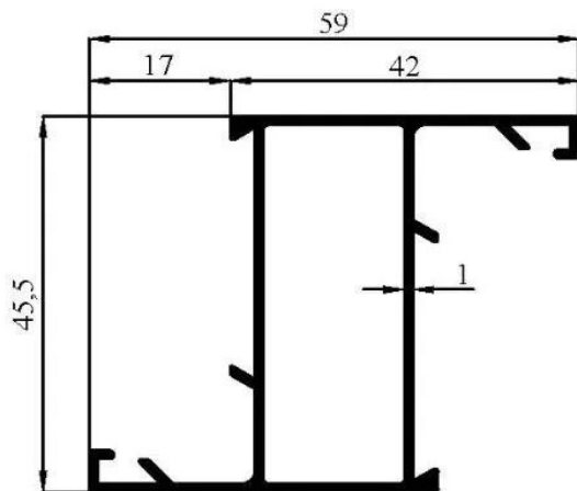
1103 0,557 kg/m
