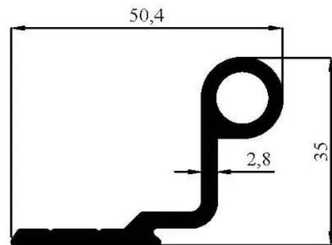
4205 0,715 kg/m
