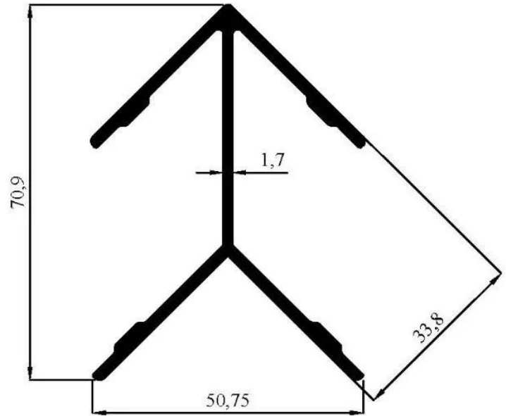
4201 1,043 kg/m
