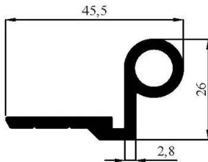
4204 0,640 kg/m
