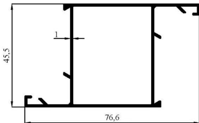
1105 0,653 kg/m
