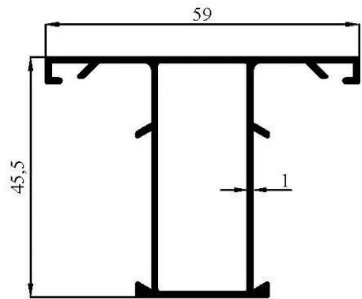
1102 0,557 kg/m
