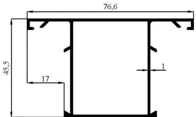
1106 0,653 kg/m
