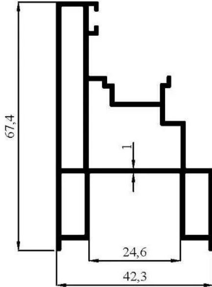
3196 0,856 kg/m
