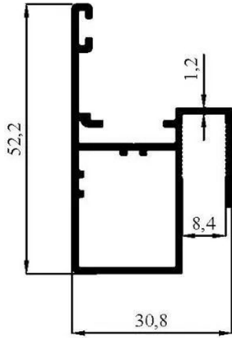
4551 0,550 kg/m
