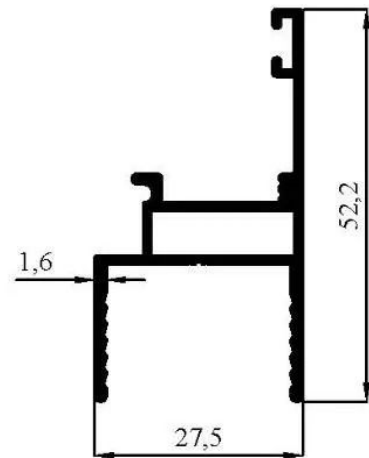
4064 0,472 kg/m
