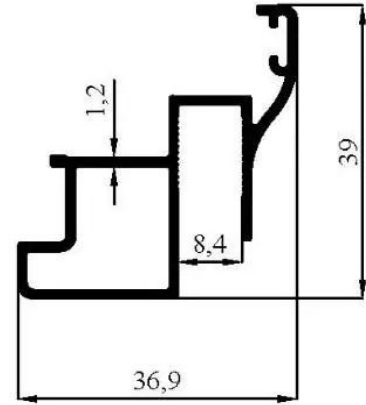
4552 0,450 kg/m
