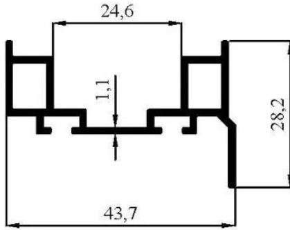
3200 0,412 kg/m
