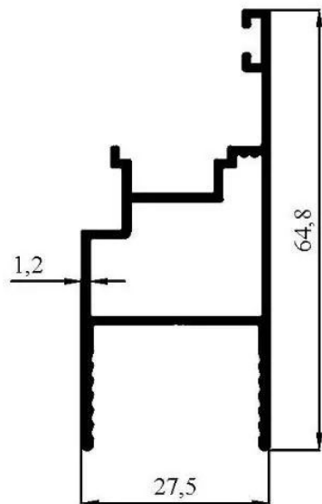
4065 0,566 kg/m
