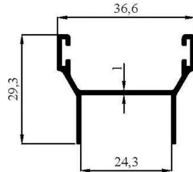
3806 0,282 kg/m
