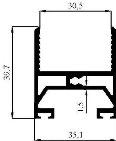
2378 0,854 kg/m
