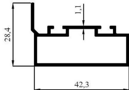
3199 0,431 kg/m
