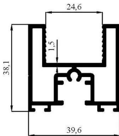
3198 0,905 kg/m
