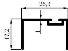
3808 0,182 kg/m
