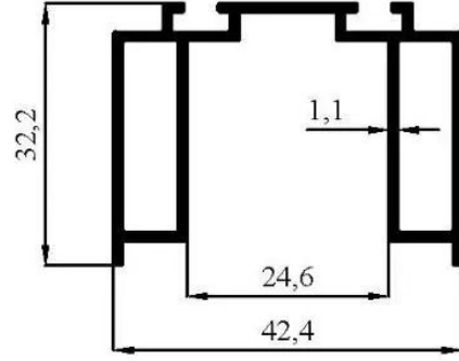
3201 0,537 kg/m
