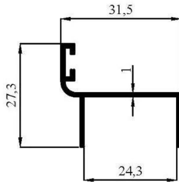
3807 0,225 kg/m
