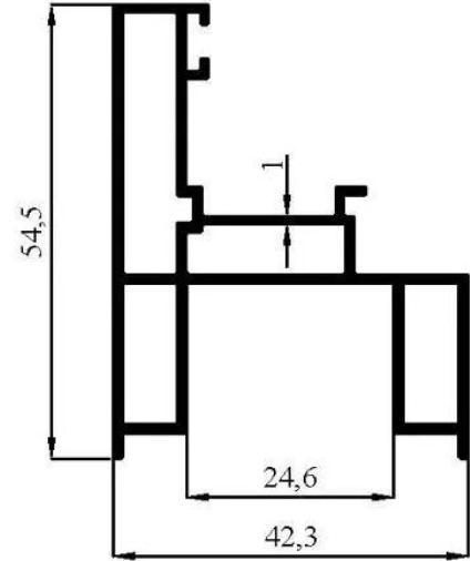
3197 0,707 kg/m
