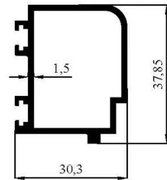
2379 0,583 kg/m
