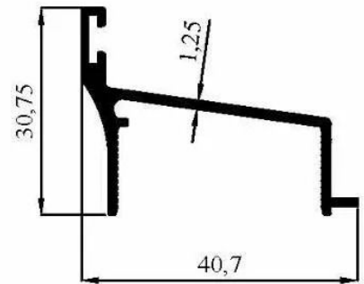
2470 0,325 kg/m
