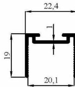
2617 0,190 kg/m
