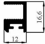
1985 0,214 kg/m
