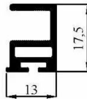
2016 0,219 kg/m
