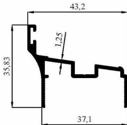
2536 0,398 kg/m
