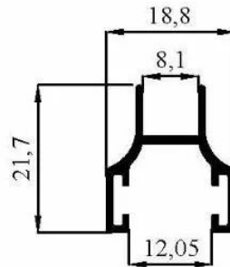
2352 0,203 kg/m
