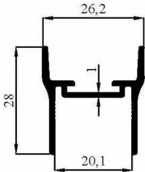
2613 0,277 kg/m
