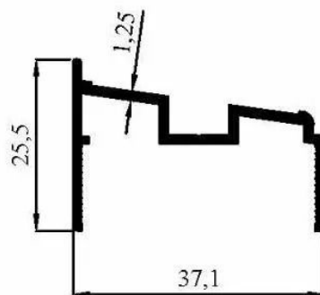
2537 0,295 kg/m
